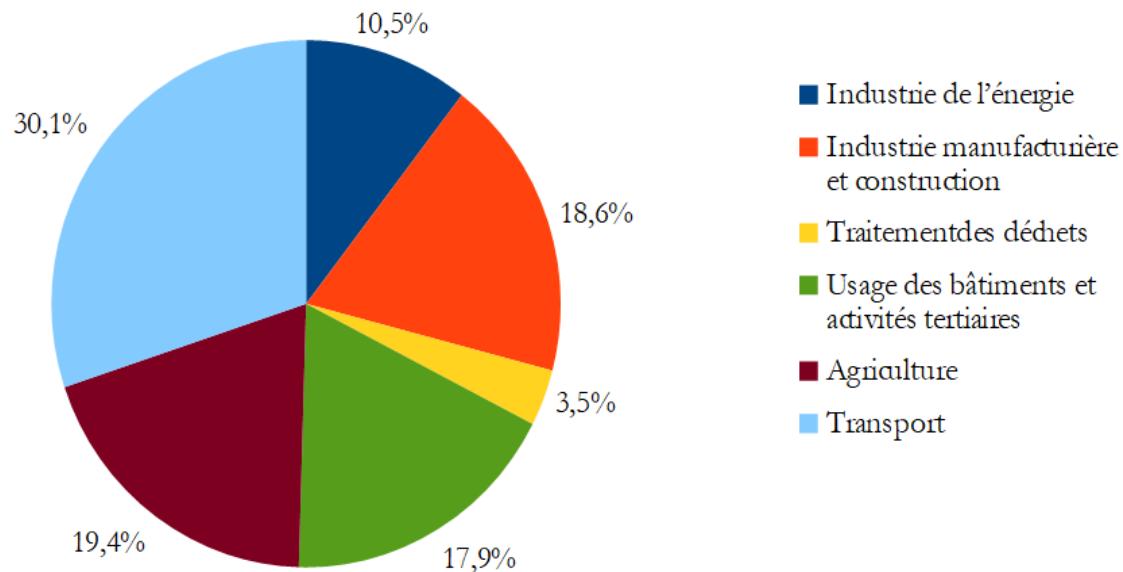
Emissions de GES dans le monde en 2021
